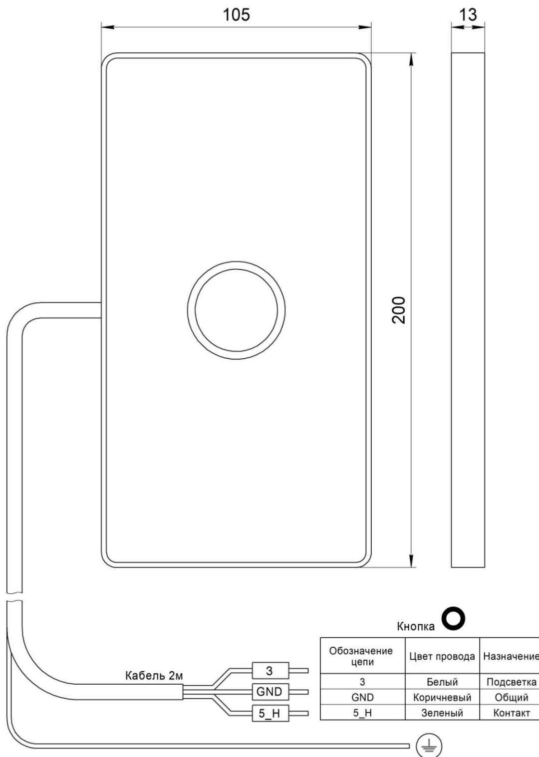
Рис.1 Внешний вид и габаритные размеры Вызывного поста МАЛАХИТ НШЕК.468381.060
